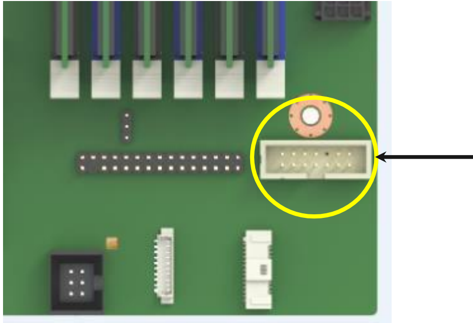
Рисунок 45. Расположение разъёма для видео на плате
