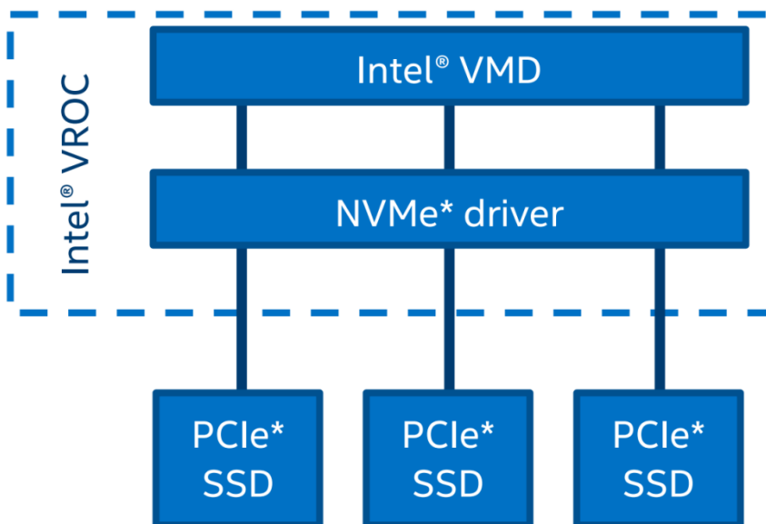
Рисунок 72. Обзор базовой архитектуры Intel® VROC
